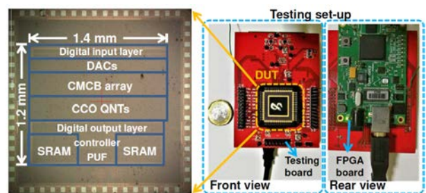
图 2 芯片显微图与测试环境图
