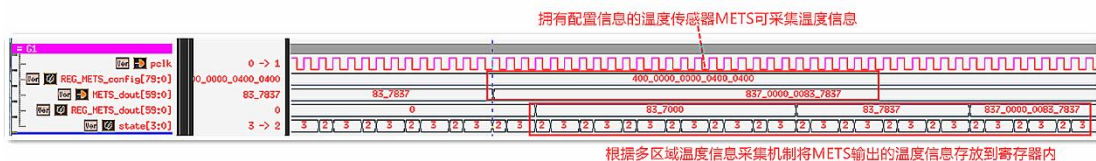
图 10 SoC 环境下 METS 配置与温度输出验证波形图
