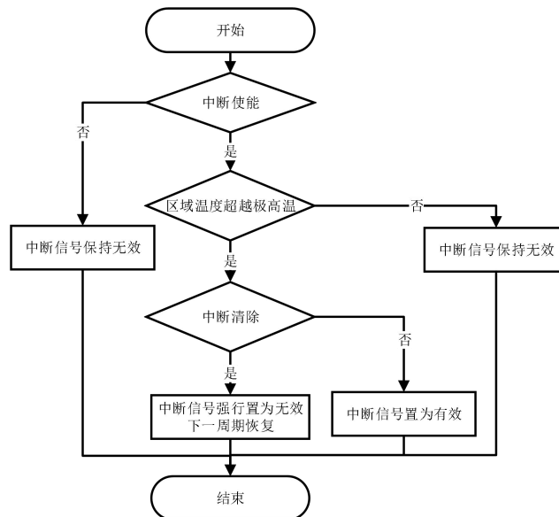
图 5 中断机制流程图
