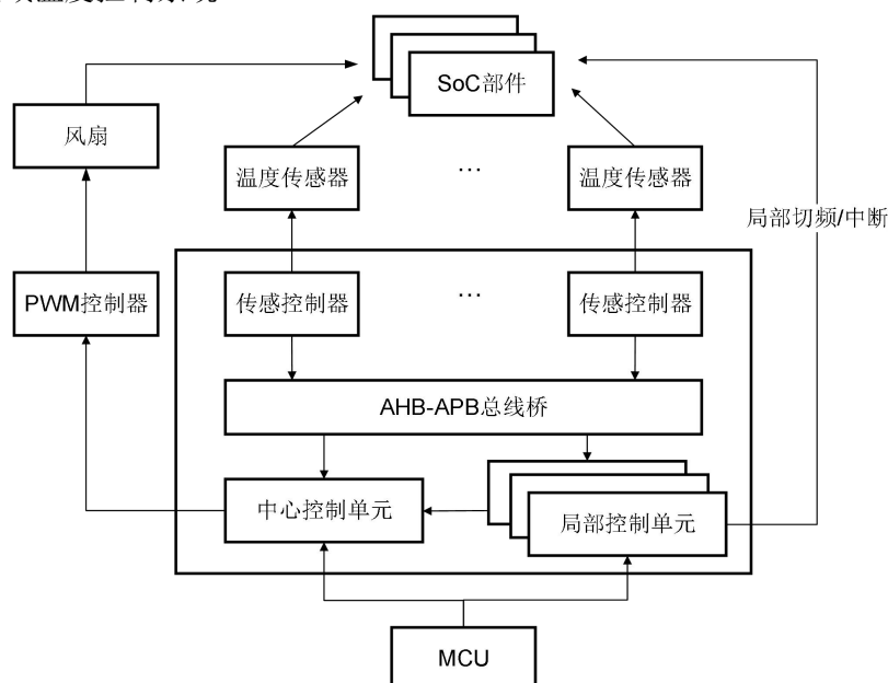
图 1 多区域温度控制系统整体架构
