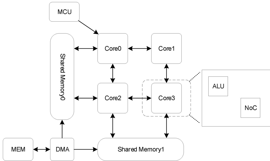
图 7 SoC 平台示意图
