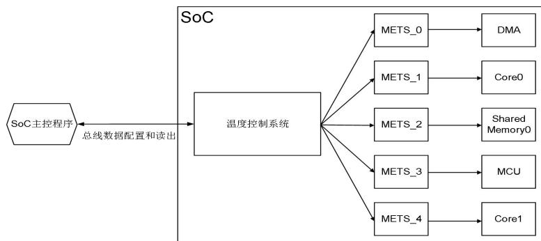
图 9 测试整体框图
