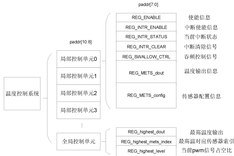
图 3 总线系统地址映射示意图
