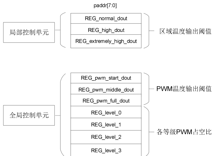
图 6 温度控制参数总线映射示意图
